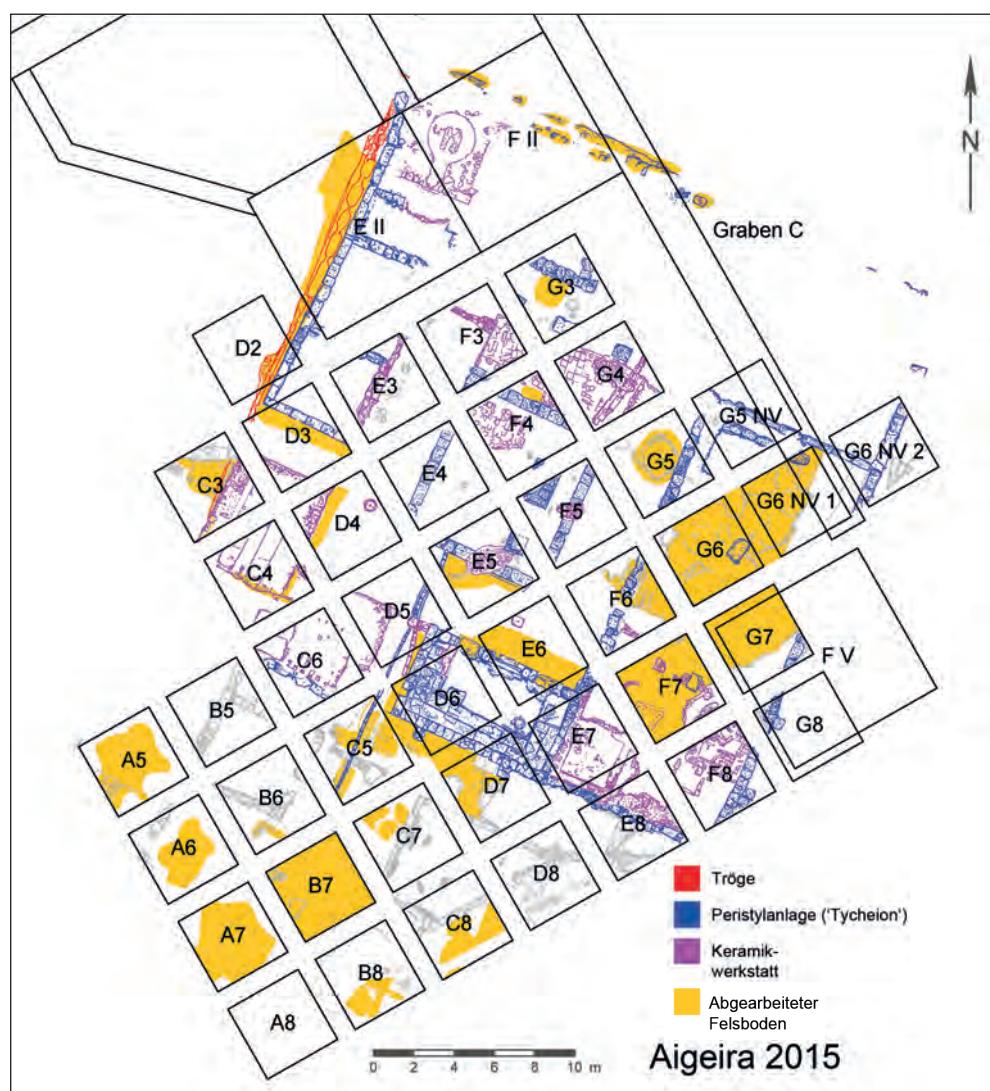
94 Phasenplan des ›Tycheions‹, gelb: abgearbeiteter Felsboden (ÖAW-ÖAI/W. Gauß – H. Birk, nach Vorlagen T. Hagn)
