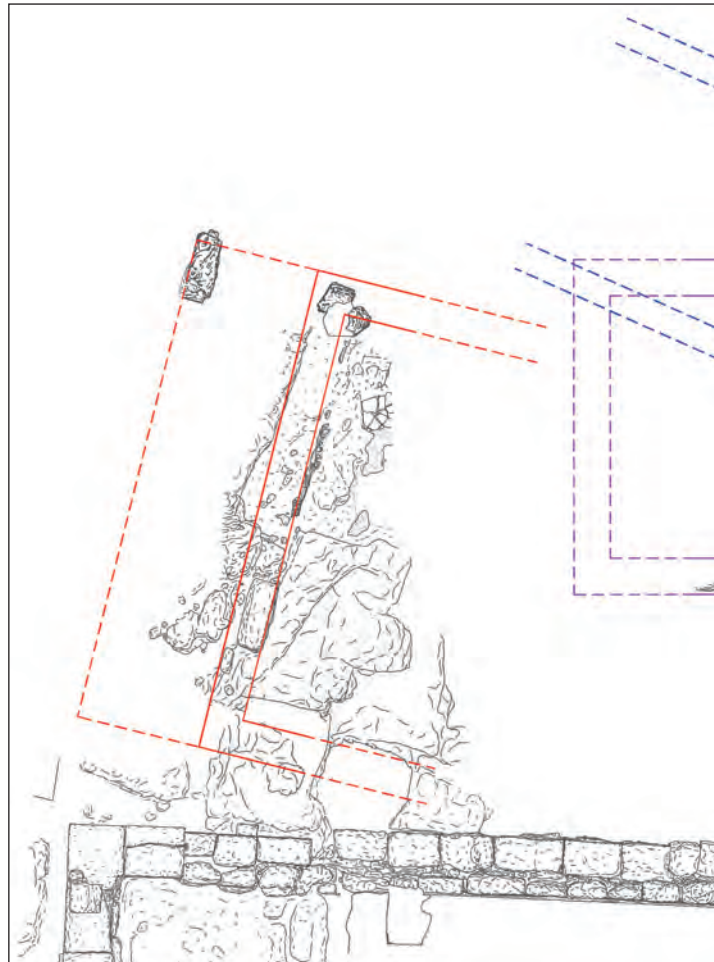
24 Grundriss von Bau C und seine Lage im Verhältnis zu Bau B und ›Naiskos‹ D (ÖAW-ÖAI/W. Gauß – H. Birk – C. Regner – A. Tanner)
