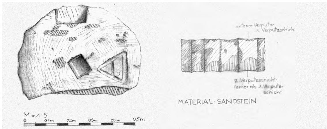
51 Säulentrommel mit Versatzmarke aus dem Podium des »Naikos« D (ÖAW-ÖAI/U. Eisenmenger)
