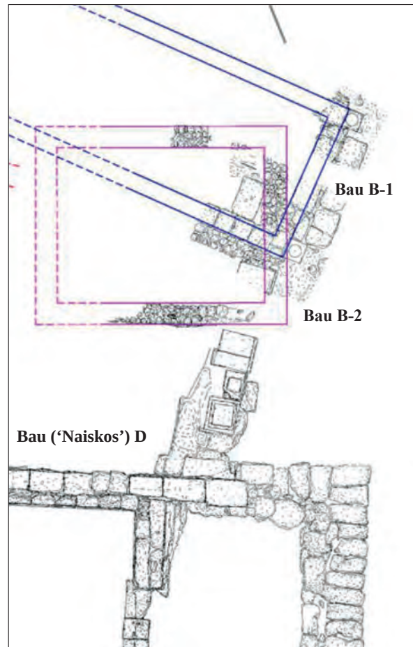
18 Bau B am Ende der Ausgrabung (jüngeres Gebäude B-2, älteres Gebäude B-1) (ÖAW-ÖAI/W. Gauß – H. Birk – C. Regner – A. Tanner)
