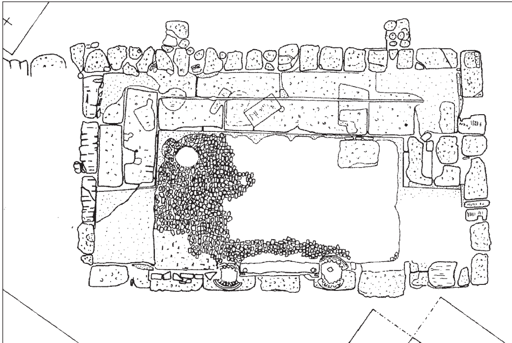
102 Grundriss der Exedra des ›Tycheions‹ (ÖAW-ÖAI/T. Hagn)
