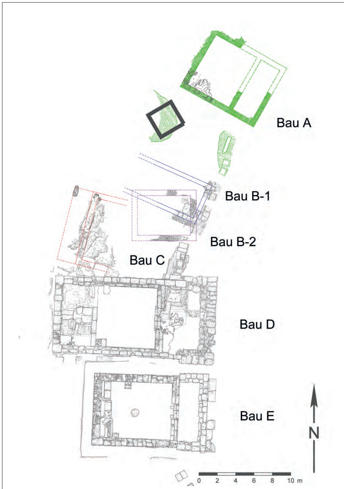
9 Bauten A–C sowie die ›Naiskoi‹ D und E, Stand 2018 (ÖAW-ÖAI/W. Gauß – H. Birk – C. Regner – A. Tanner). Die grün hervorgehobenen Abschnitte wurden von O. Walter freigelegt.
