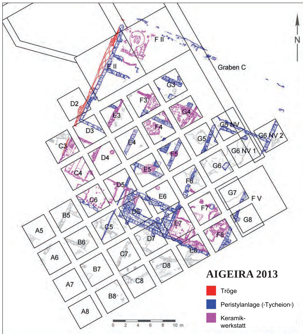
88 Phasenplan des ›Tycheions‹ (ÖAW-ÖAI/W. Gauß – H. Birk nach Vorlagen von W. Alzinger – T. Hagn)
