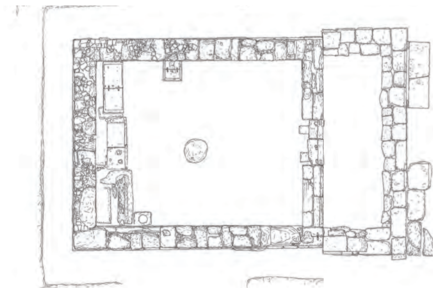
53 Grundriss des ›Naiskos‹ E (ÖAW-ÖAI/A. Tanner)
